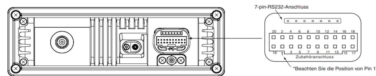
Abbildung 17 Position des Zubehöranschlusses und des Erweiterungsanschlusses – Rückseite
