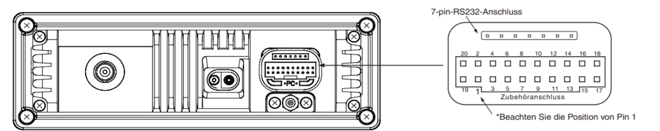
Abbildung 17 Position des Zubehöranschlusses und des Erweiterungsanschlusses – Rückseite
