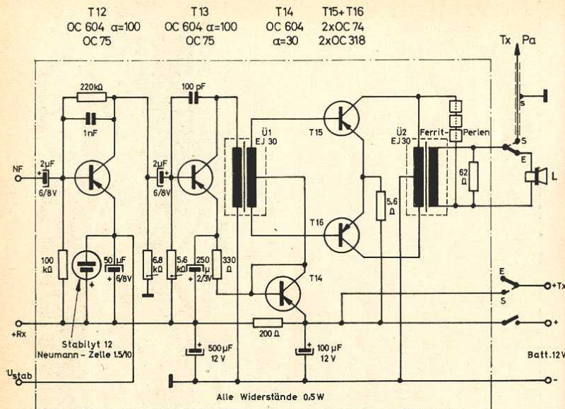
Abb.9: Modulator bzw. NF - Verstärker DL 6 SW (Schaltung)
