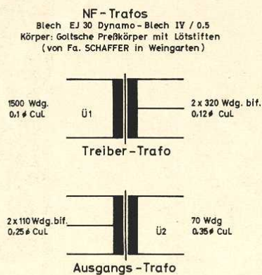
Abb.10: Übertrager für Modulator bzw. NF - Verstärker DL 6 SW
