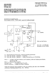
Anschlussvorschlag VFO
