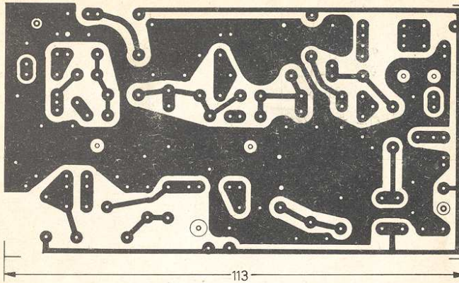
Abb. 2 a Leiterseite
