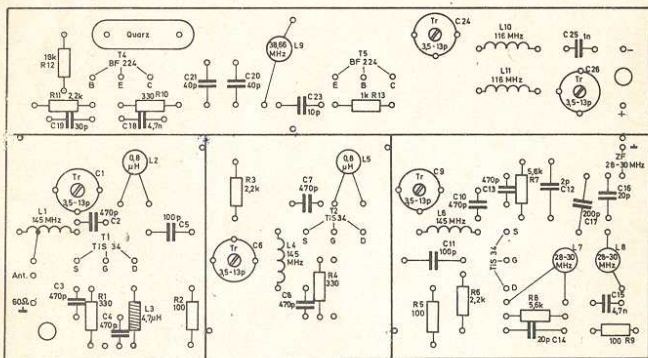
Abb. 2 b Bestückungsplan
