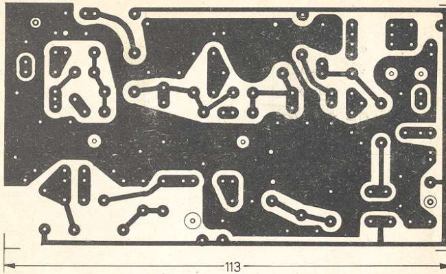
Abb. 2 a Leiterseite
