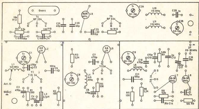
Abb. 2 b Bestückungsplan
