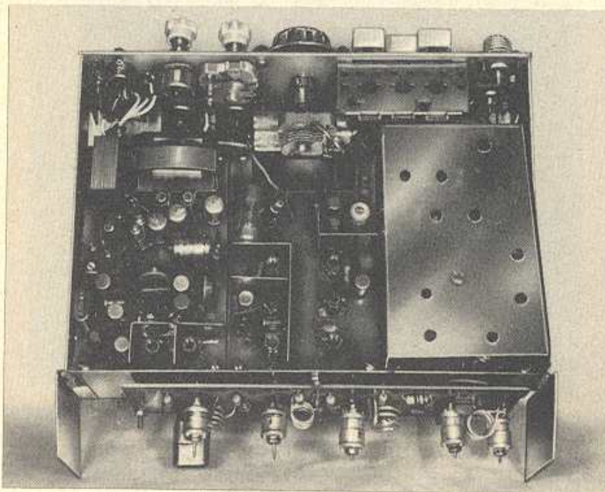
Bild 92. Innenansicht der 2-m-Station von DL 9 IW
