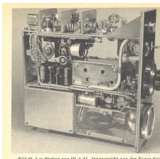
Bild 87. 2-m-Station von DL 9 AL, Innenseite von der Tuner-Seite
