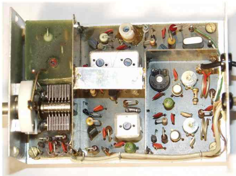
Abb. 1 Blick von oben in das Teko- -Gehäuse des 2 H 71 MO. Links auf der Platine die Kam- mer des VFOs, oben rechts der Festoszillator mit seinem Quarz. In der Mitte neben der Ab- schirmwand der Trimmer für die Output-Regelung, R 25, und C 30 für die Einstellung der Auskopp- lung. In der VFO-Kammer erkennt man deutlich die vergossenen, frequenzbestimmenden Teile so- wie den sehr stabilen Drehkon- densator.
