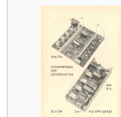
Zusammenbau Leiterplatten
