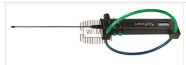
Peilempfänger mit Rahmenantenne
