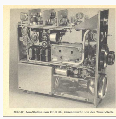
2m Station von DL9AL , Tunerteil
