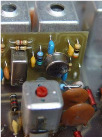
Zusatzplatine auf dem Konvert
