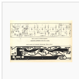
Empfänger Leiterplatte
