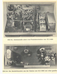
Innenansicht der DJ5MM 2m Transistorstation
