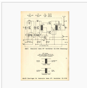
Modulator Nf- Verstärker
