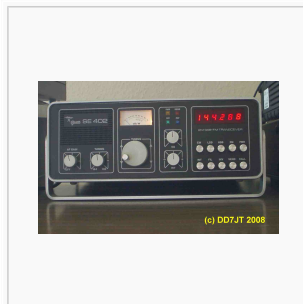
Tischgerät SE 402, FM, SSB, CW; Pout: 10 W (1977)
