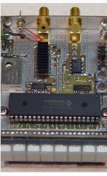
Frequenzzähler, von Gabor Gesce
