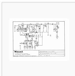
Hael AM/FM Sender Schaltbild
