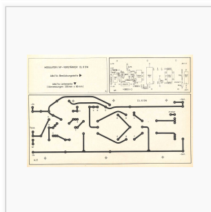
Modulator, NF Verstärker
