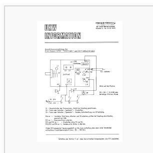
Anschlussvorschlag VFO
