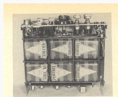
Kleine Transistorstation von DL9AL
