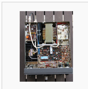
HG74A Unterseite
