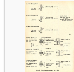
Empfänger Schaltbild
