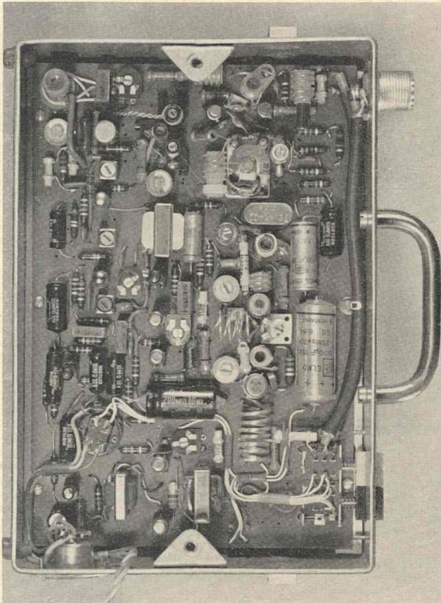
Abb. 4 Funksprechgerät „Trausnitz III“ offen von hinten (Bestückungsseite der Leiterplatte)
