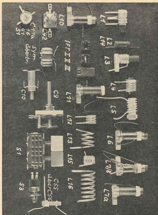
Abb. 11 Spulen, Bandfilter und verschiedene Bauteile für das Funksprechgerät „Trausnitz III“
