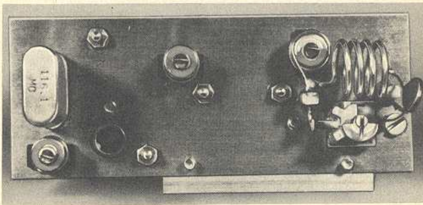
Bild 82. Der Senderbaustein aus der Station von DJ 5 MM von oben gesehen
