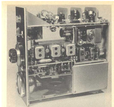
Bild 88. Innenaussicht der 2-m-Station von DL9AL mit Zf-Baustein
