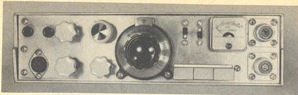
Bild 91. Frontansicht der 2-m-Transistorstation von DL 9 IW
