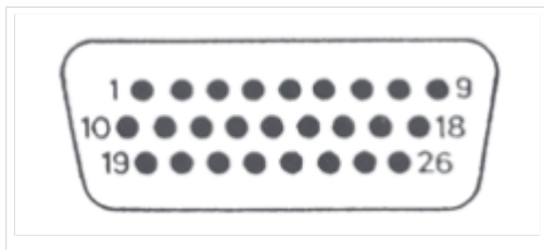
Sub-D 26 Pin des Hytera Repeaters
