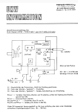
Anschlussvorschlag VFO
